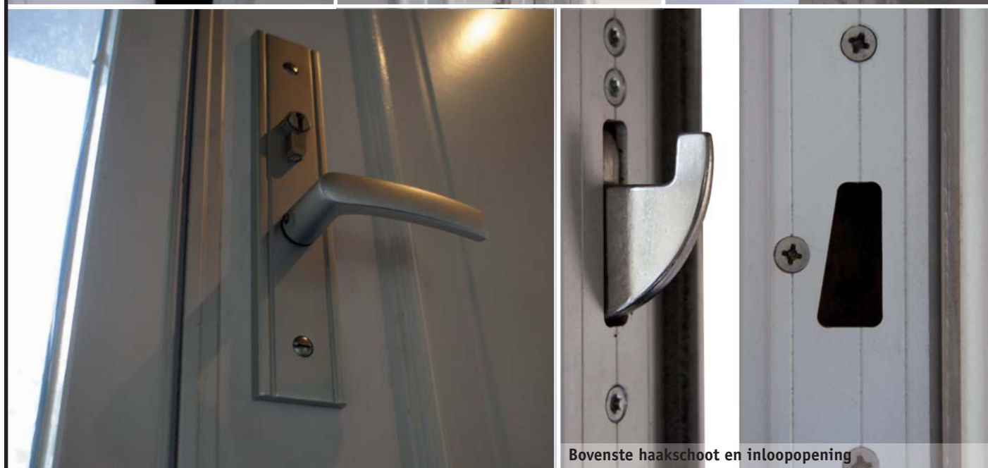
Inloopening voor de haakschoot en dagschootsparing.
