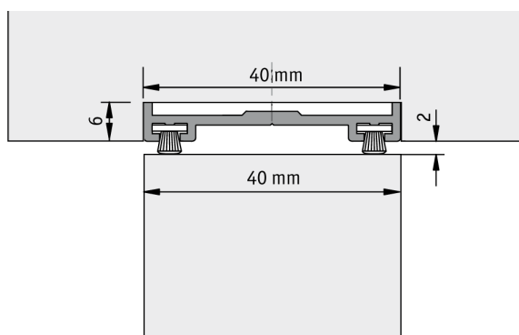
Afbeelding 2. Technische tekening, doorsnede
